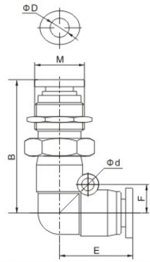
SPLM系列隔板直角 SPML Series—Bulkhead Union Elbow
