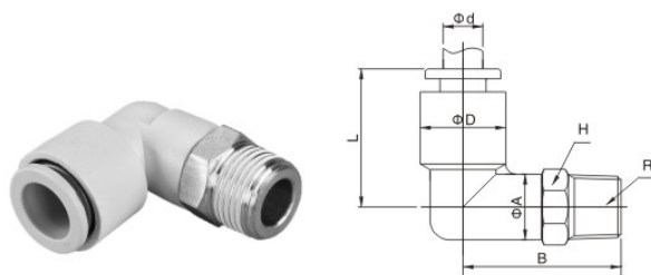
KQ2L 系列-螺纹弯通 KQ2L Series-Male Elbow
