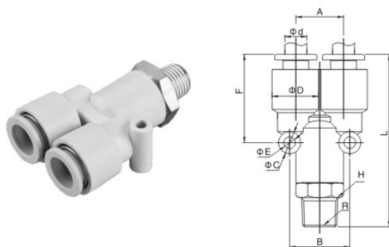
KQ2X 系列-Y型螺纹三通 KQ2X Series-Male "Y"
